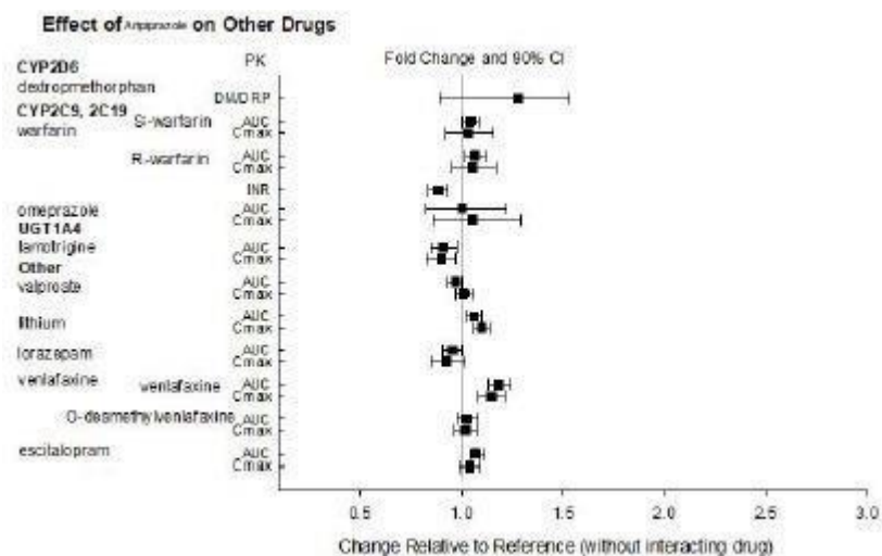
圖 3：aripiprazole對其它藥物的藥動學作用
