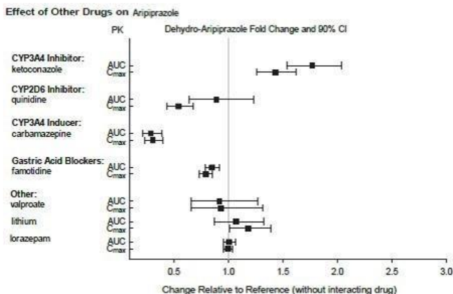
圖 2：其它藥物對dehydro-aripiprazole的藥動學作用
